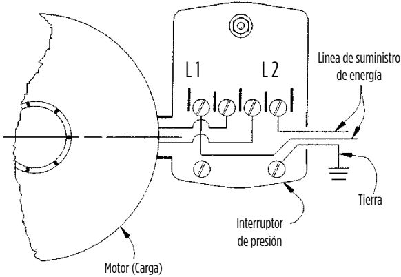
Fig. 10 – CONEXIONES ELÉCTRICAS
