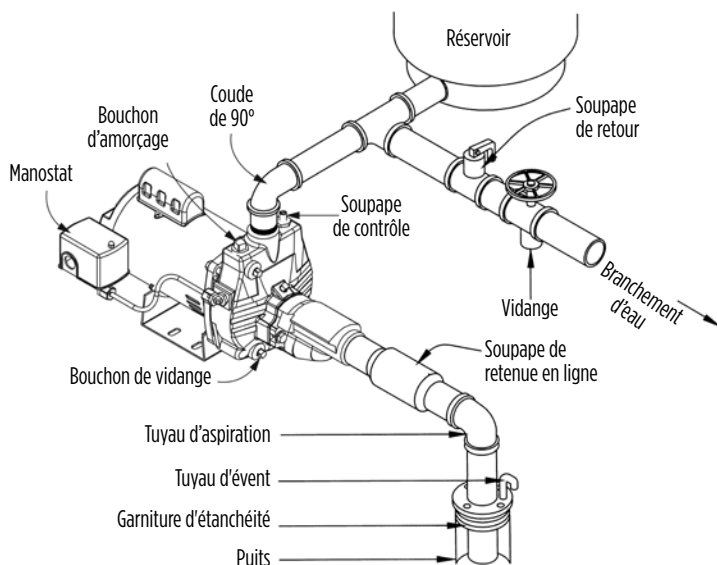
Illustr. 9b - PUITS PEU PROFOND (avec soupape de retenue en ligne)
