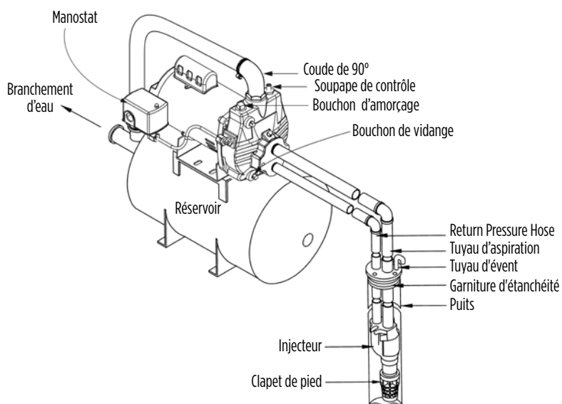
Illustr. 9d - PUITS PEU PROFOND - SYSTÈME MONTÉ SUR LE RÉSERVOIR (avec clapet de pied)
