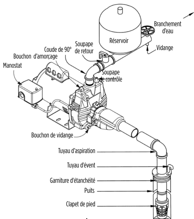
Illustr. 9c - PUITS PEU PROFOND - RÉSERVOIR EN LIGNE (avec clapet de pied)
