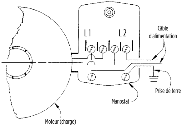
Illustr. 10 - BRANCHEMENTS ÉLECTRIQUES
