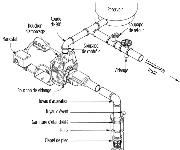
Illustr. 9a - PUITS PEU PROFOND (avec clapet de pied)
