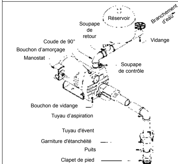
Fig. 4c PUIITS PEU PROFOND - RÉSERVOIR EN LIGNE (AVEC CLAPET DE PIED)
