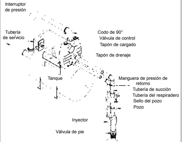
Fig. 4d POZO PROFUNDO - SISTEMA MONTADO EN EL TANQUE (INSTALACIÓN CON TUBERÍA DOBLE CON VÁLVULA DE PIE)
