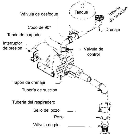
Fig. 4c POZO POCO PROFUNDO - TANQUE EN LA LÍNEA (CON VÁLVULA DE PIE)
