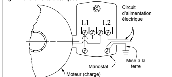
Fig. 2 Branchements électriques
