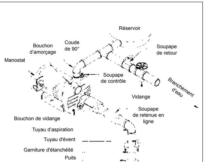
Fig. 4b PUIITS PEU PROFOND (AVEC SOUPAPE DE RETENUE EN LIGNE)
