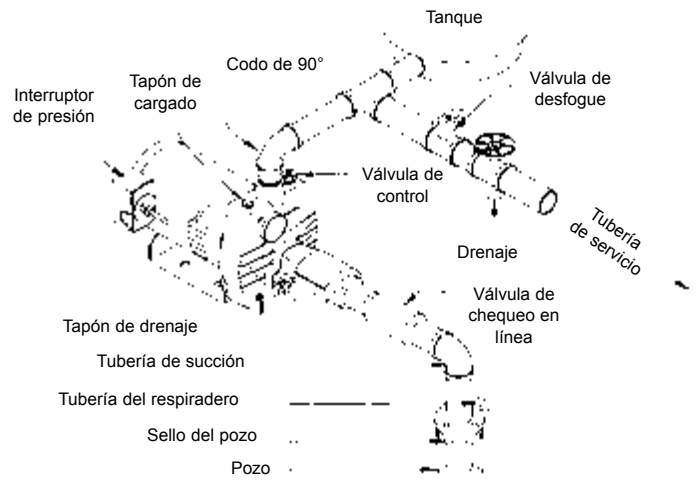
Fig. 4b POZO POCO PROFUNDO (CON VÁLVULA DE CHEQUEO EN LÍNEA)
