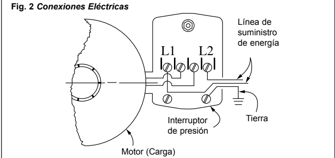
Fig. 2 Conexiones Eléctricas
