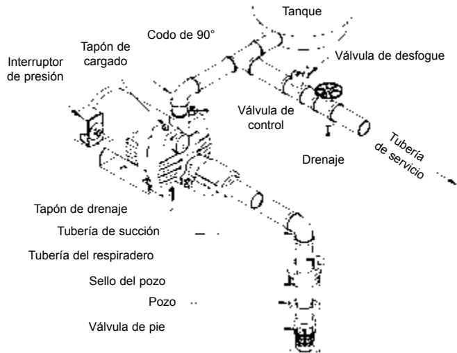
Fig. 4a POZO POCO PROFUNDO (CON VÁLVULA DE PIE)
