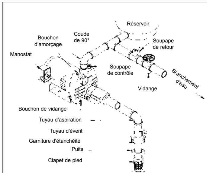
Fig. 4a PUIITS PEU PROFOND (AVEC CLAPET DE PIED)
